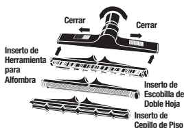
Boquilla maestra de plástico ABS de 35,56cm (14")
