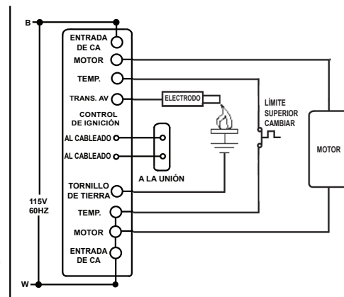
DIAGRAMA ESQUEMÁTICO
