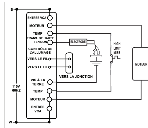
DIAGRAMME SCHEMATIQUE
