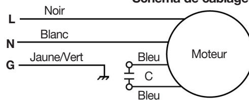
Schéma de câblage
