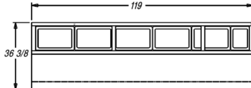
DP119 TOP
