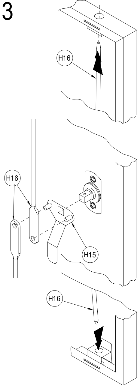
RIGHT DOOR ROD ASSEMBLY
