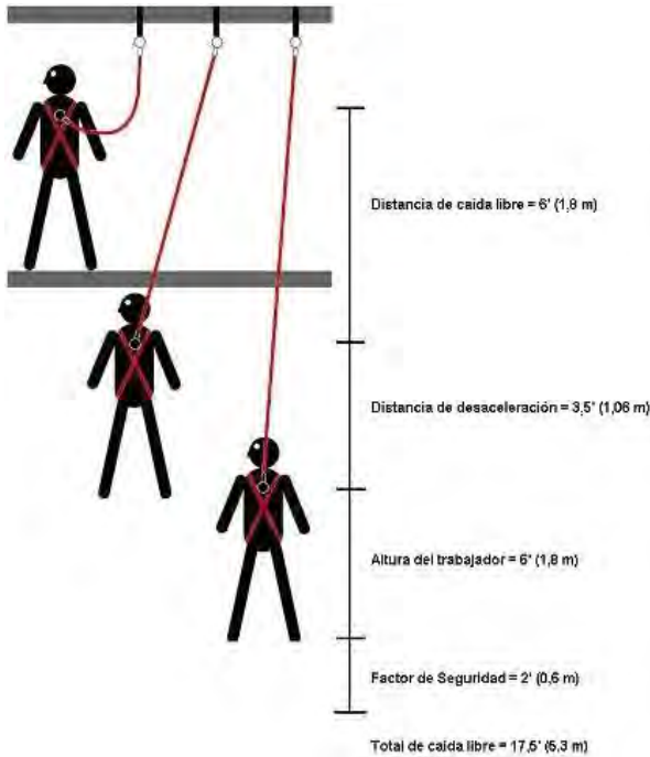
Figura 2.1: Diagrama de caída despejada
